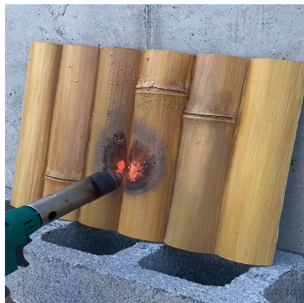
不燃素材やけず竹（不焼竹）燃焼試験
