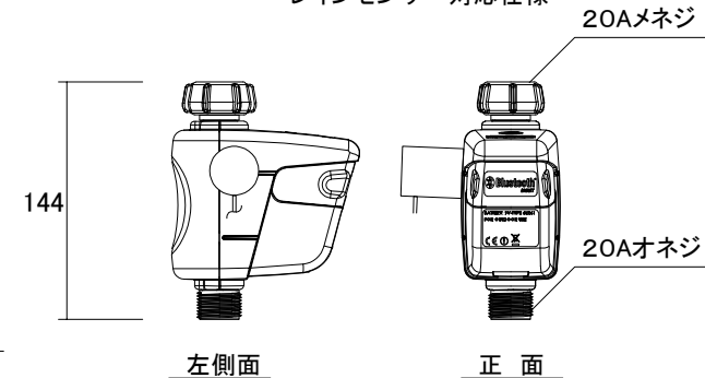
左側面
