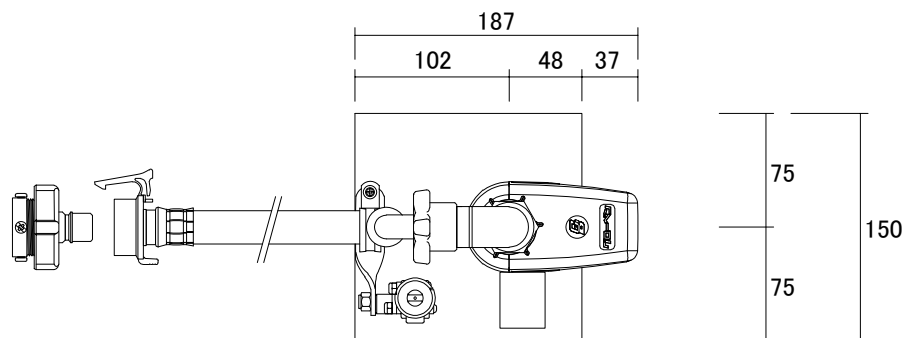
平面
