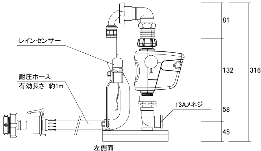
左側面
