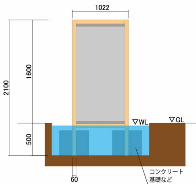
基本セットA（水中自立型）
