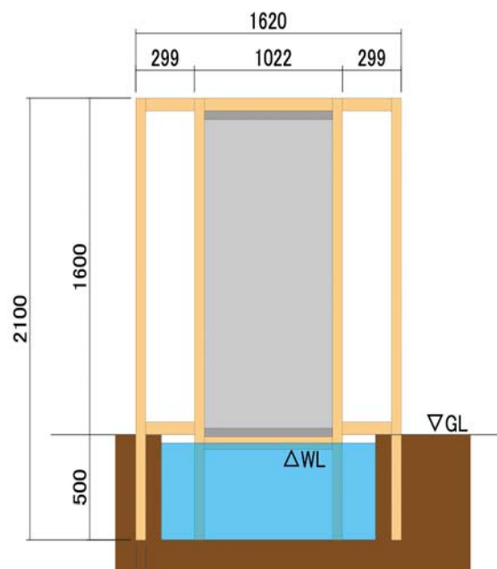
基本セットB（陸上埋設型）
